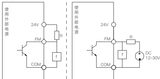
图 4-9 FM 端子接线
